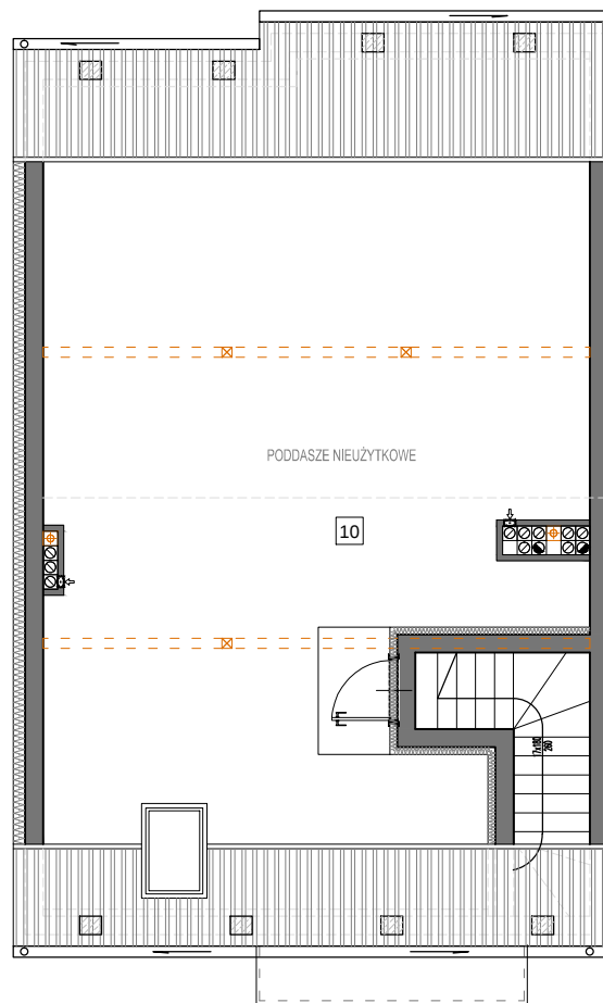
plan poddasza
